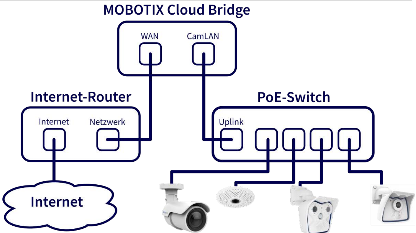
Abb. 1: Verbindungsschema für die MOBOTIX Cloud Bridge
